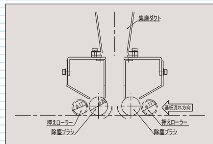
除塵ローラー部断面図
